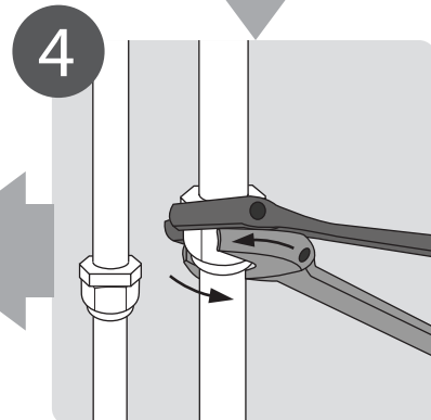
4 Присоедините трубы хладагента
