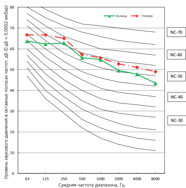
M4OB-36HFN8-Q
