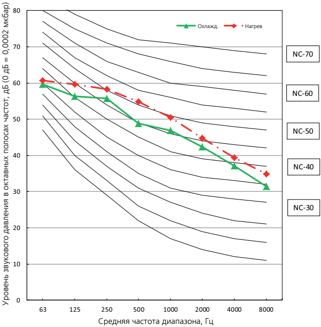
M2OG-14HFN8-Q
