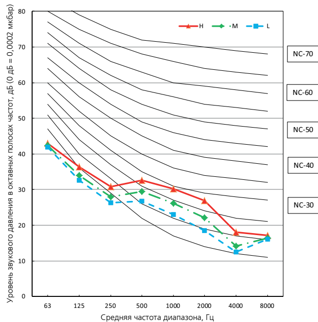
MTIU-12NXD0
