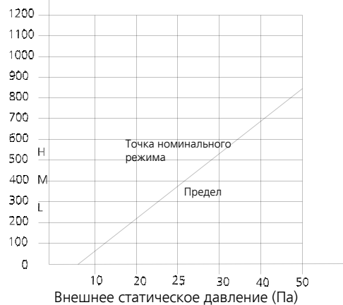
Объемный расход воздуха (м³/ч) SP3
