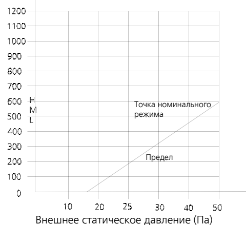
Объемный расход воздуха (м³/ч) SP4 PS: SP4 M==SP3 H
