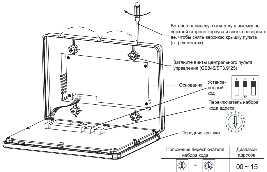
Рисунок 1.2. Монтажная схема
