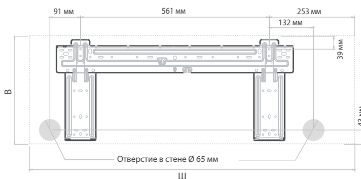
Размеры внутреннего блока (Ш×В): 968 мм x 322 мм
