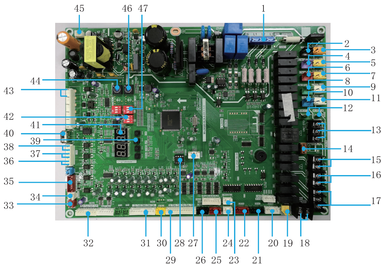
Рисунок 8-11. Главная плата моделей MCDH82A-PR3 и MCDH164A-PR3
