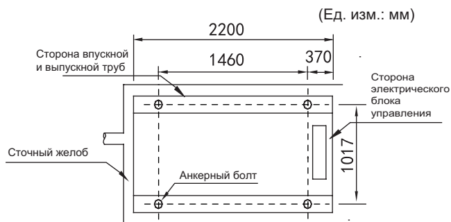
Рисунок 6-7. Вид сверху на схематический чертеж с монтажными размерами моделей MCDH82A-PR3 и MCDH130A-PR3
