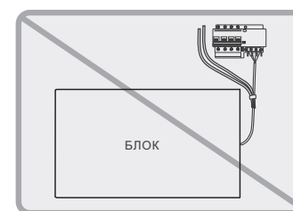
Рисунок 8-24-3. Система управления и меры предосторожности при монтаже (с)
