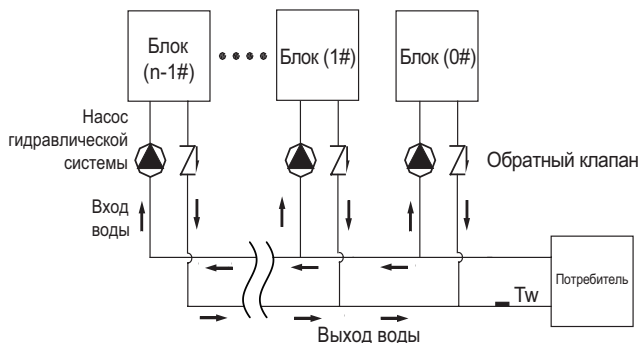
Рисунок 8-34. Монтаж нескольких насосов гидравлической системы
