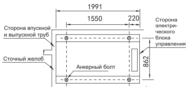
Рисунок 6-6. Вид сверху на схематический чертеж с монтажными размерами модели MCDH70A-PR3
