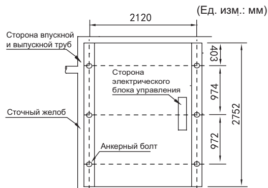
Рисунок 6-8. Вид сверху на схематический чертеж с монтажными размерами модели MCDH164A-PR3
