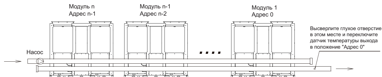
Рисунок 8-32. Установка нескольких модулей (не более 8) MCDH164A-PR3
