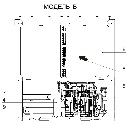
Рисунок 8-3. Основные элементы модели MCDH130A-PR3 (рисунок приведен только для иллюстрации взаимного расположения основных элементов)
