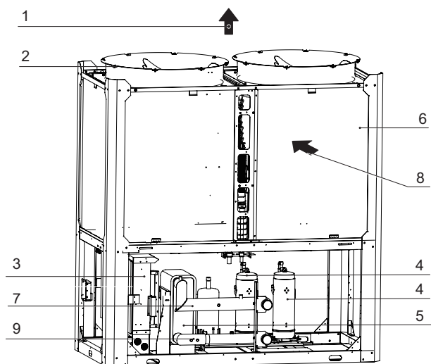
Рисунок 8-3. Основные элементы модели MCDH130A-PR3 (рисунок приведен только для иллюстрации взаимного расположения основных элементов)
