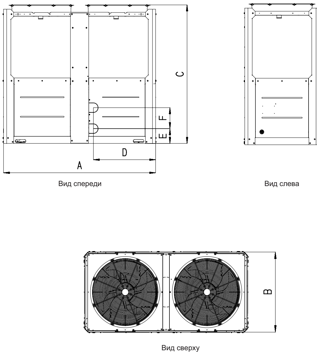
Рисунок 6-1. Габаритный чертеж
