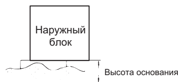
Рисунок 6-11. Высота основания для защиты от снега
