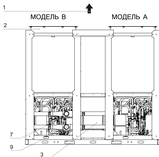
Рисунок 8-4. Основные элементы модели MCDH164A-PR3 (рисунок приведен только для иллюстрации взаимного расположения основных элементов)
