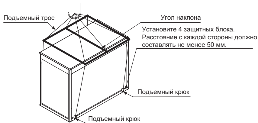
Рисунок 3-1. Подъем чиллера
