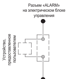
Рисунок 8-23. Подключение разъема «ALARM»
