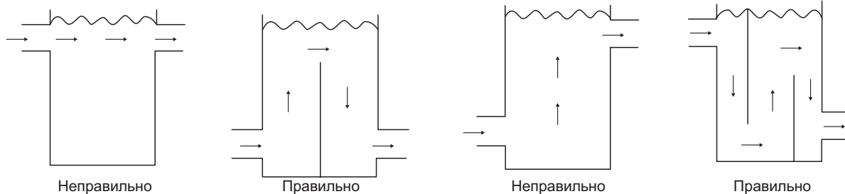
Рисунок 8-26. Конструкция накопительного бака
