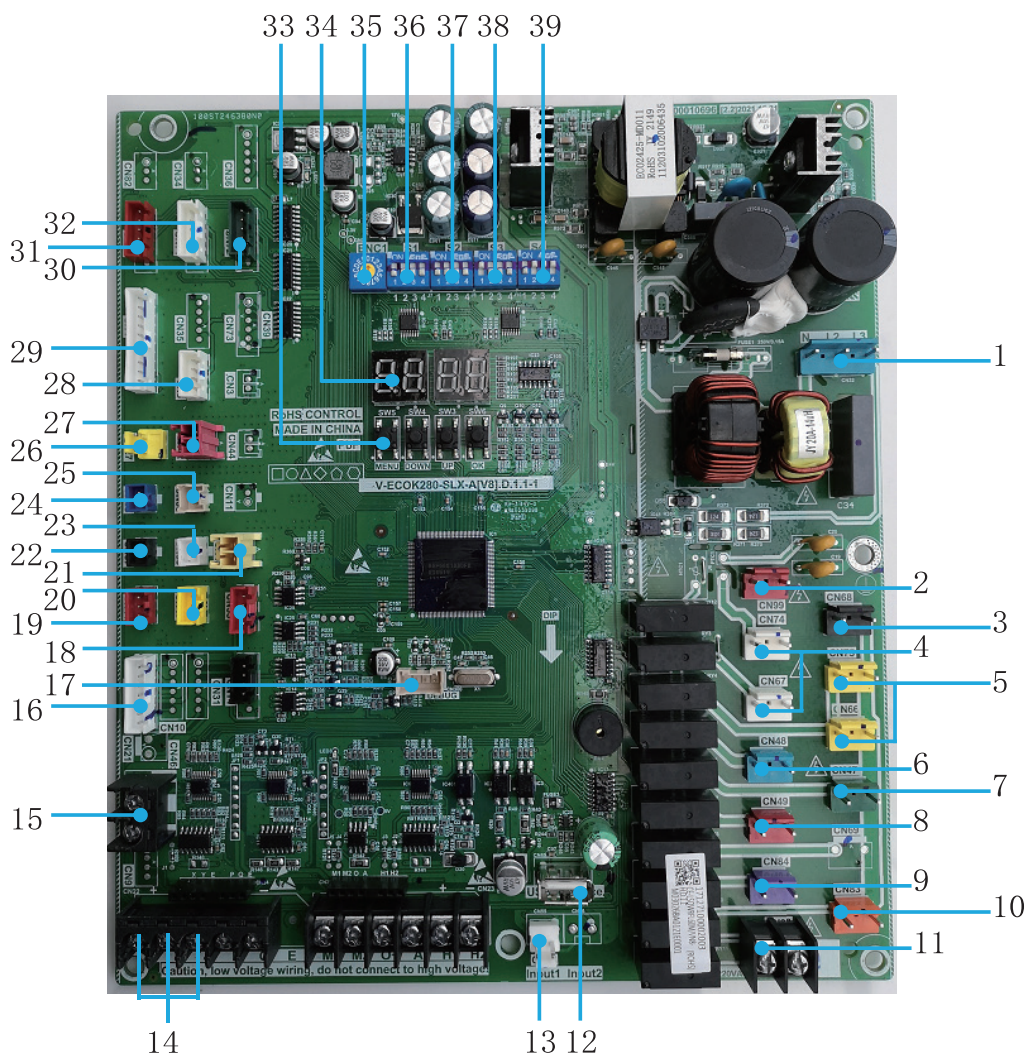
Рисунок 8-9. Главная плата моделей MCDH70A-PR3 и MCDH130A-PR3
