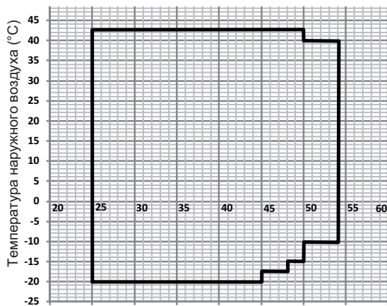
Температура воды на выходе (°C) Рисунок 1-1-2 Диапазон рабочих температур в режиме нагрева
