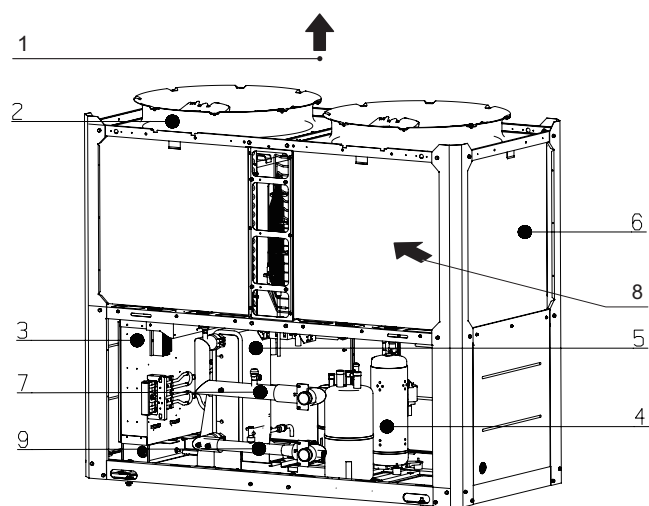
Рисунок 8-1. Основные элементы модели MCDH70A-PR3 (рисунок приведен только для иллюстрации взаимного расположения основных элементов)
