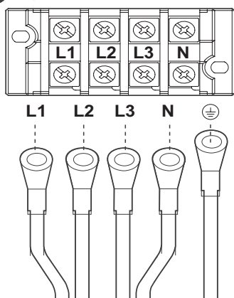
Рисунок 8-17 Требования к подключению силовой электропроводки
