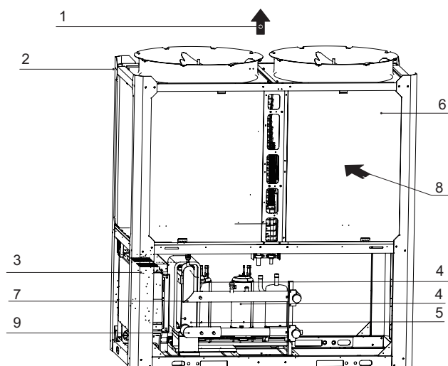
Рисунок 8-2. Основные элементы модели MCDH82A-PR3 (рисунок приведен только для иллюстрации взаимного расположения основных элементов)
