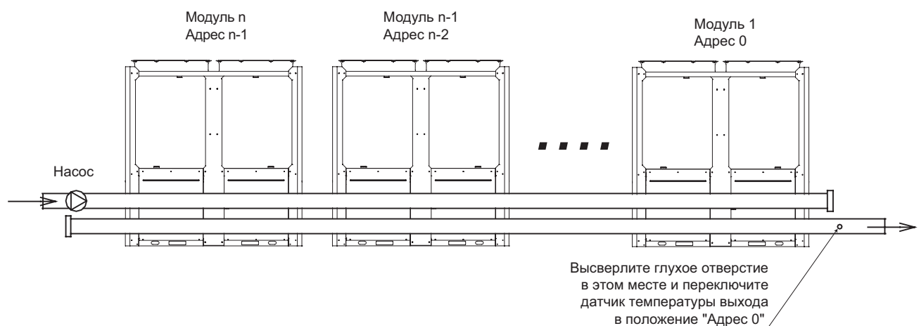
Рисунок 8-31. Установка нескольких модулей (не более 16)
