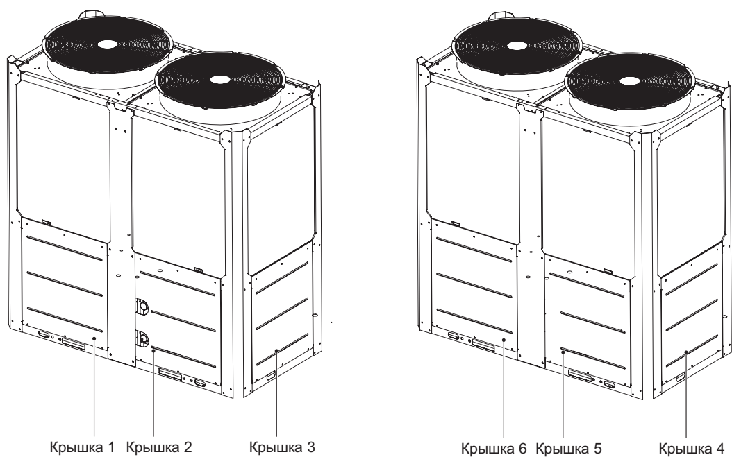
Рисунок 8-6. Дверцы модели MCDH70A-PR3
