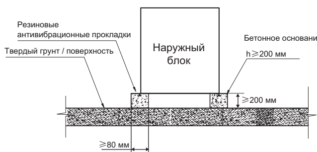
Рисунок 6-5. Вид спереди на конструкцию основания
