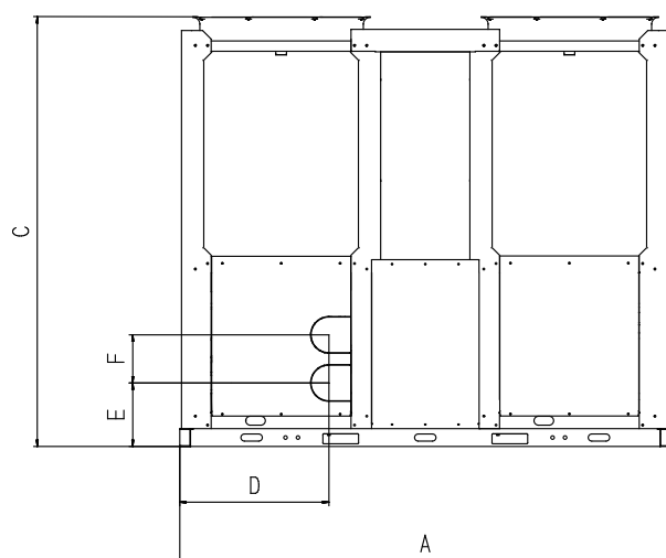
Вид спереди
