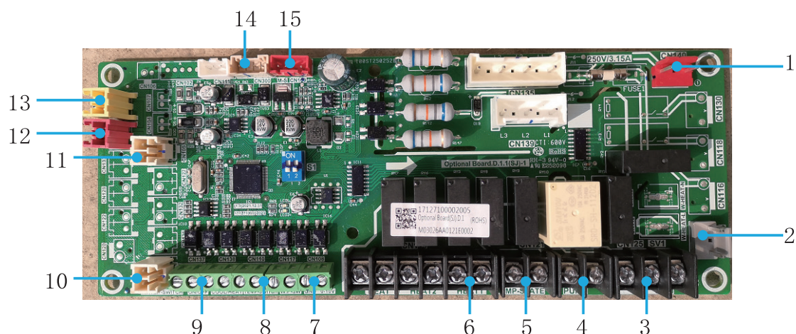
Рисунок 8-10. Ведомая плата моделей MCDH70A-PR3 и MCDH130A-PR3
