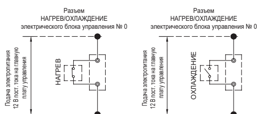
Рисунок 8-21-2. Подключение слаботочного разъема переключения НАГРЕВ/ОХЛАЖДЕНИЕ
