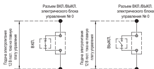
Рисунок 8-21-1. Подключение слаботочного разъема включения и выключения
