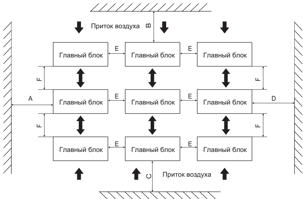
Рисунок 6-4. Монтаж нескольких блоков
