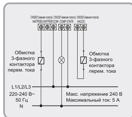
Рисунок 8-20. Схема электропроводки насоса гидравлической системы, вспомогательного нагревателя трубопровода и светового индикатора перем. тока состояния компрессора (только для моделей MCDH82A-PR3 и MCDH164A-PR3)
