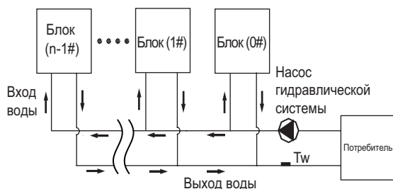
Рисунок 8-33 Монтаж одного насоса гидравлической системы
