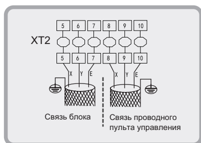
Рисунок 8-18. Подключение кабелей связи устройства и проводного пульта управления
