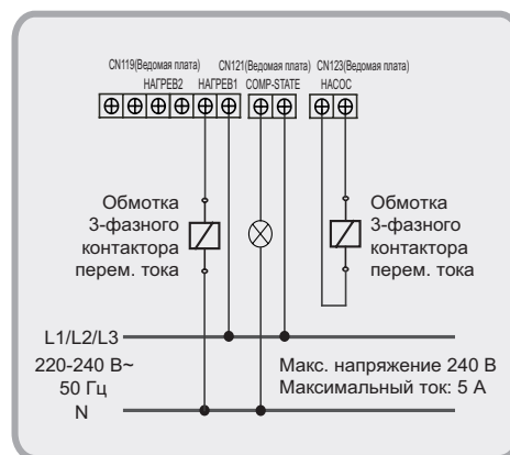
Рисунок 8-19. Схема электропроводки насоса гидравлической системы, вспомогательного нагревателя трубопровода и светового индикатора перем. тока состояния компрессора (только для моделей MCDH70A-PR3 и MCDH130A-PR3)
