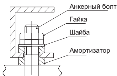
Рисунок 6-9. Установка амортизатора
