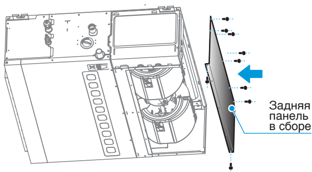
Монтаж задней панели
