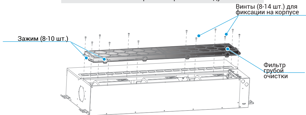
Блок с задним забором возвратного воздуха
