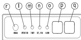
Панель управления и индикации внутреннего блока
