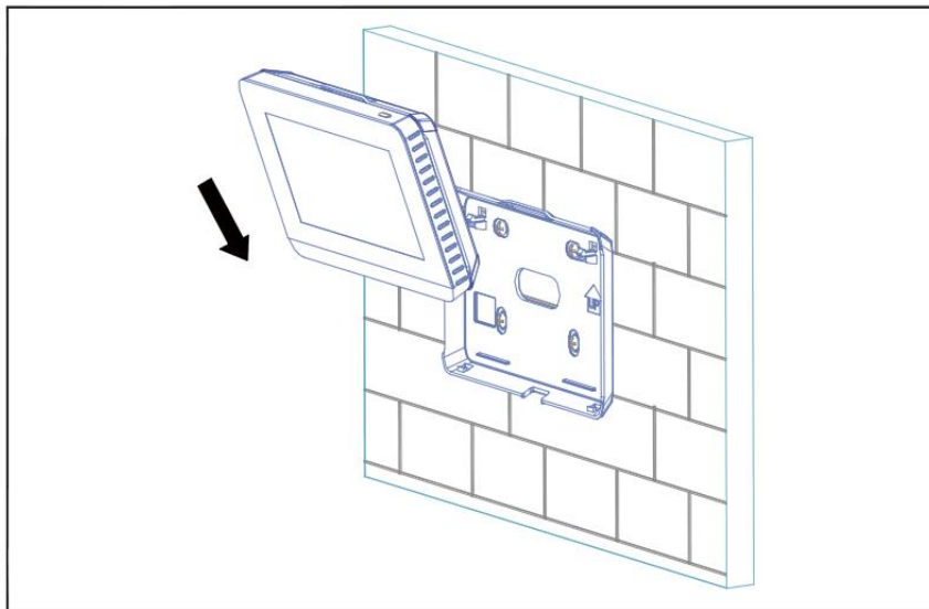
Рис.5 Вставьте пульт в крышку
