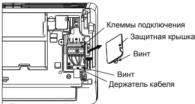
Клеммы для подключения проводов на внутреннем блоке
