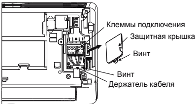
Для моделей 12 и 18 Клеммы 1,2(N) и заземление - 1,5 мм(2) клеммы 3 и 4 - 0,75 мм(2)
