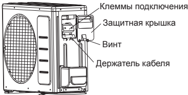
Клеммы для подключения проводов на наружном блоке
