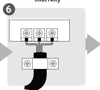
Подключите электропроводку
