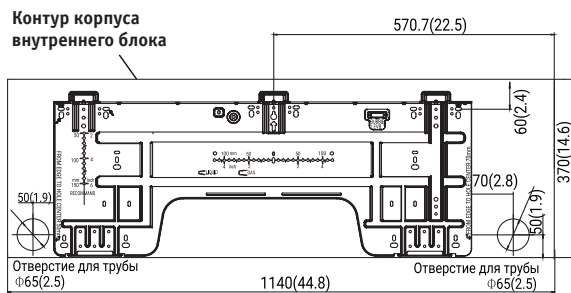
Типоразмер С
