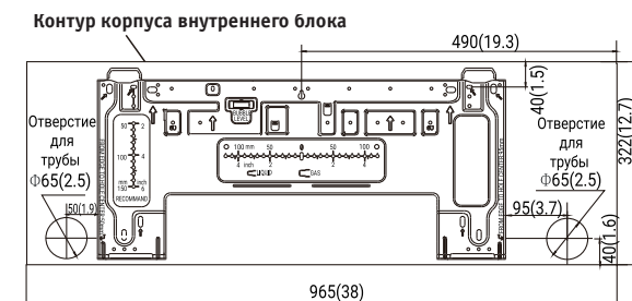
Типоразмер В
