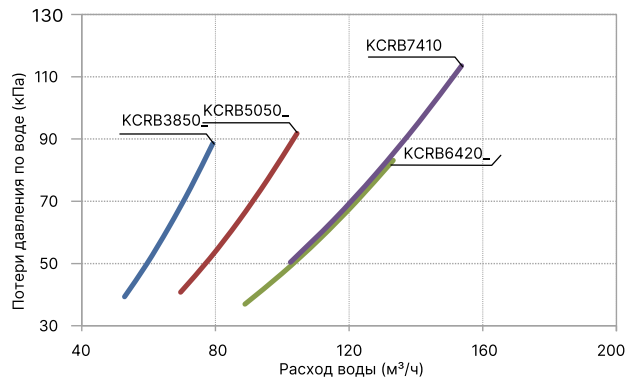
KCRB_CWCN3
