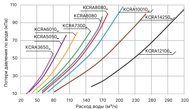
KCRA_CWCN3
