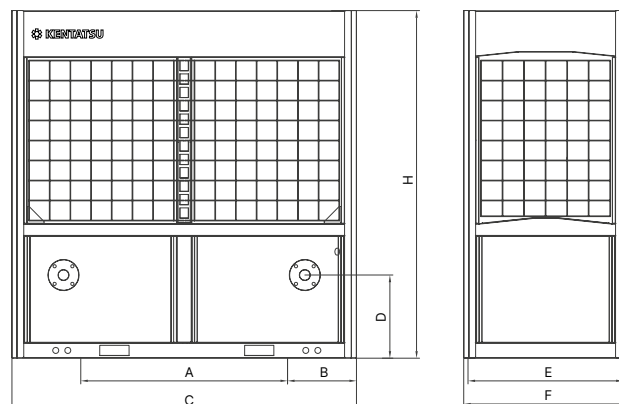
KCRN650-1300HZAN3A
