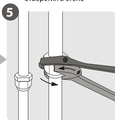
Соедините трубы
