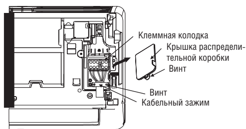
Клеммная колодка наружного блока
