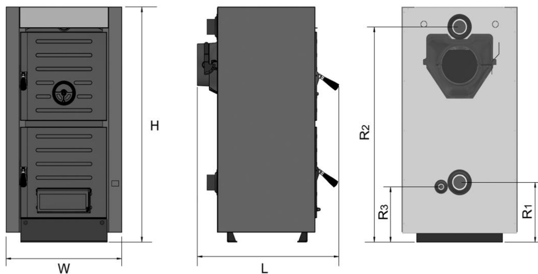
Рис. 14. Размеры котла
