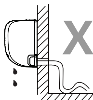
НЕПРАВИЛЬНО
