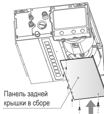
Монтаж панели задней крышки в сборе
