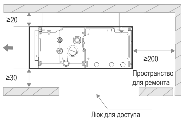
Вид сбоку
