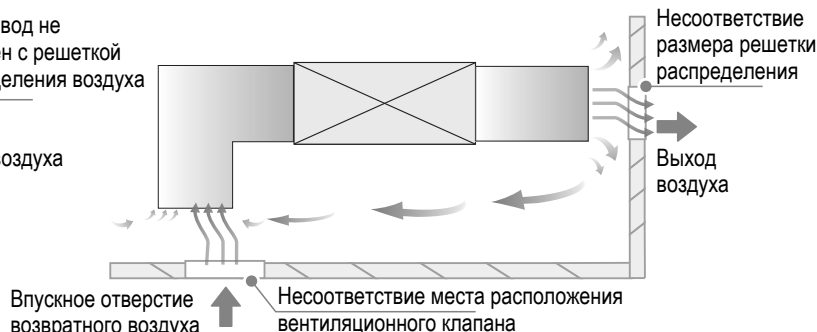
Несоответствие размера и места расположения вентиляционного клапана
