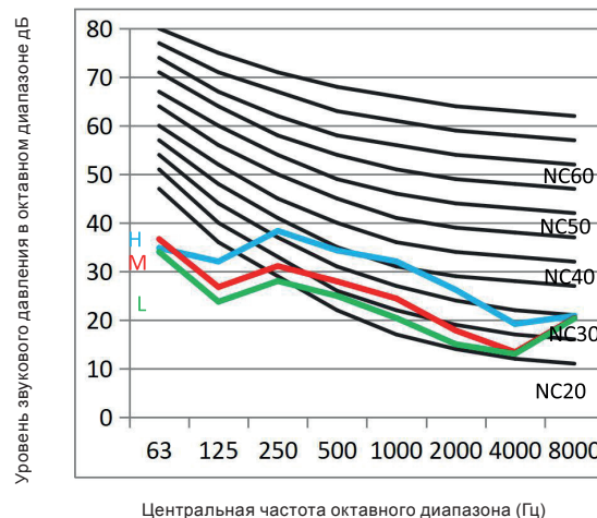
Уровни звукового давления в октавных полосах частот КТКА50НQAN1
