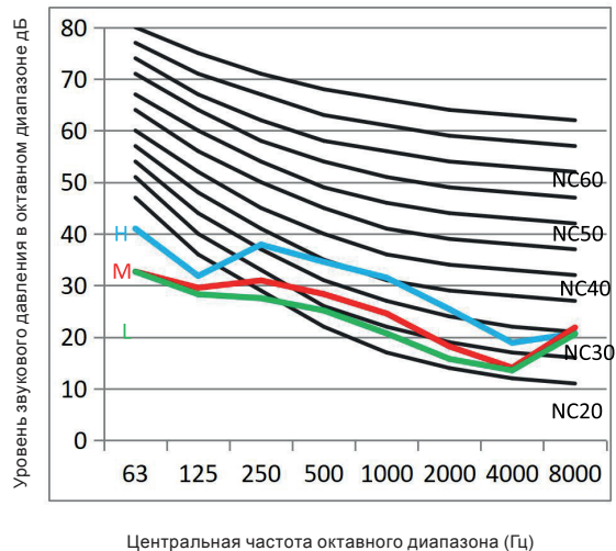
Уровни звукового давления в октавных полосах частот КТКА60НQAN1
