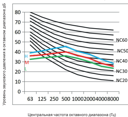
Уровни звукового давления в октавных полосах частот КТКА115НQAN1
