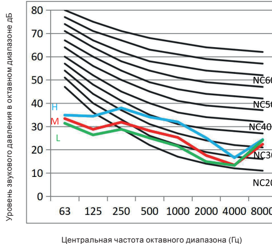
Уровни звукового давления в октавных полосах частот КТКА72НQAN1
