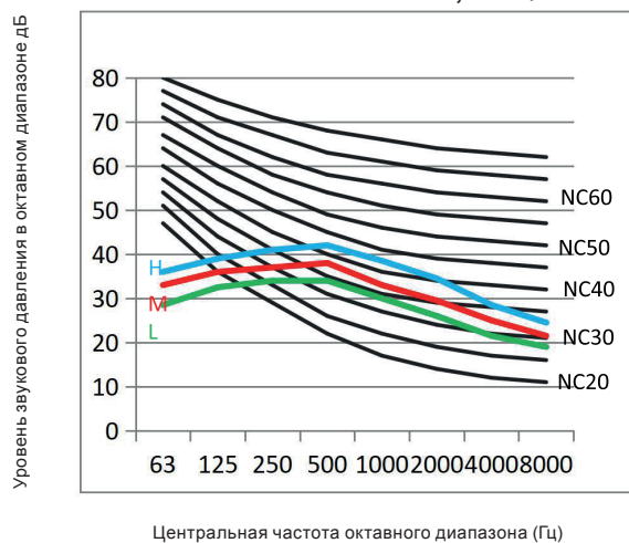
Уровни звукового давления в октавных полосах частот КТКА80,90НQAN1
