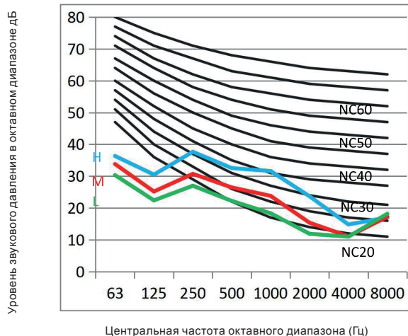
Уровни звукового давления в октавных полосах частот КТКА40НQAN1
