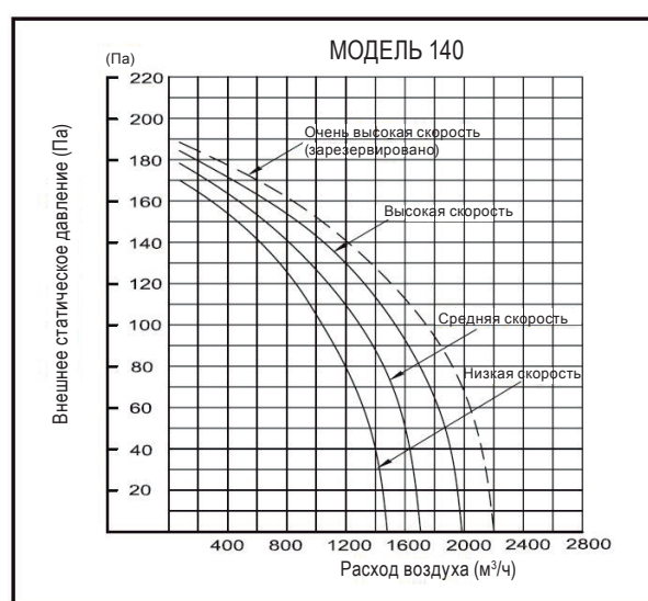
График рабочих характеристик блоков
