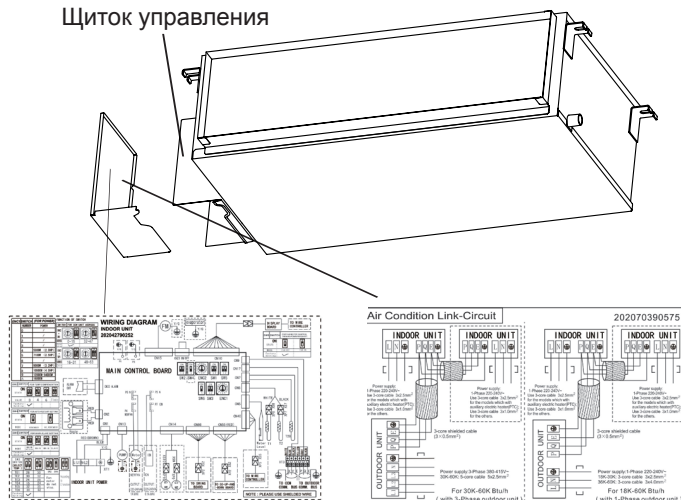
Электрическая схема
