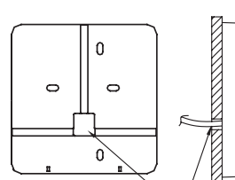
Установочное отверстие в стене и отверстие для кабеля. Диаметр отверстия в стене 2 см
