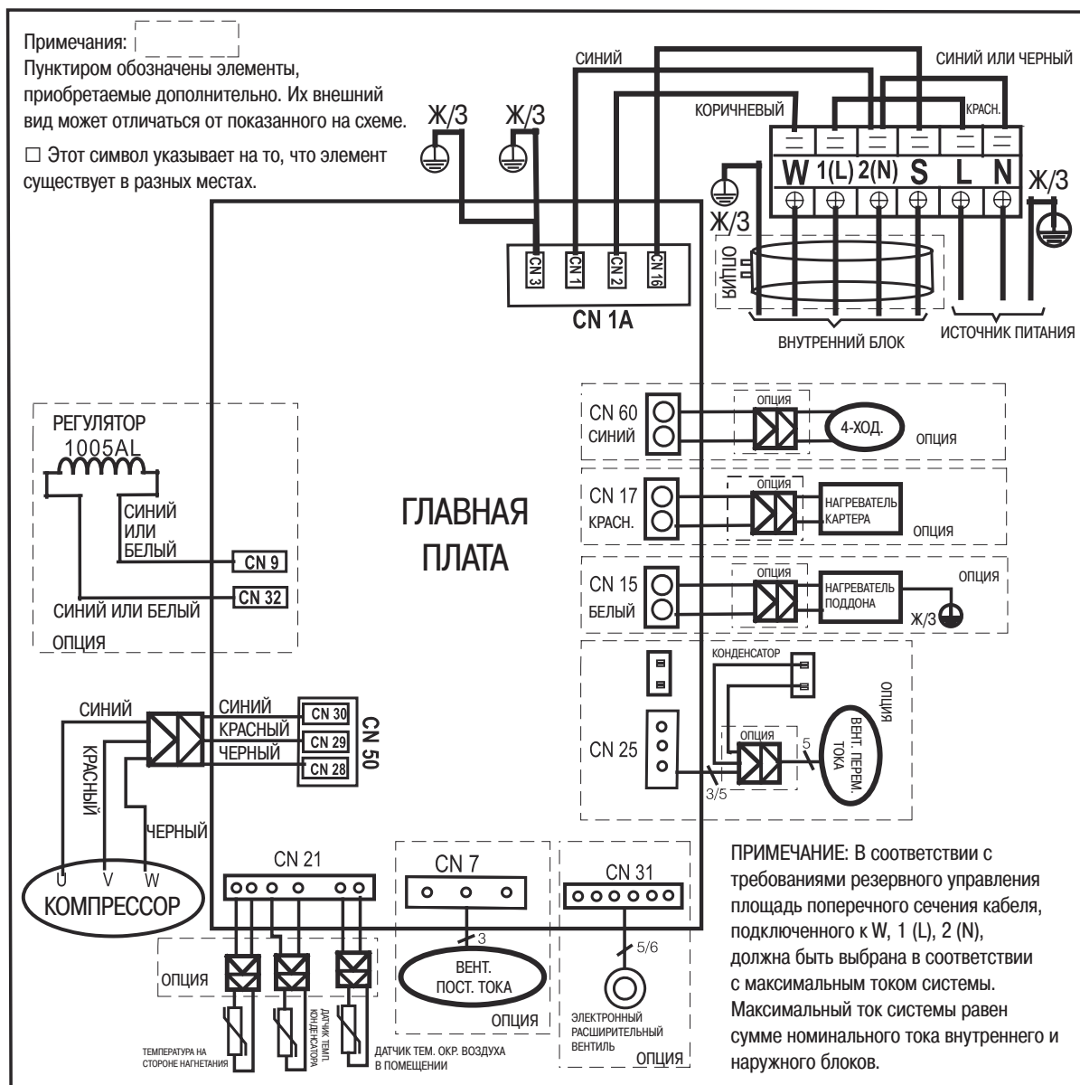
Схема электропроводки наружного блока: KSRA53HZRN1
