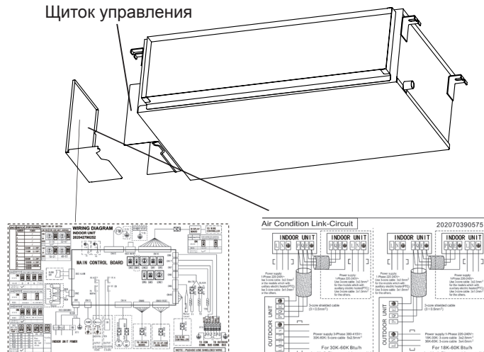
Электрическая схема
