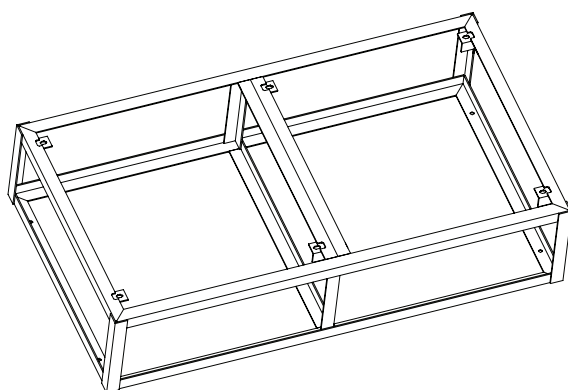
Общий вид и размеры монтажной рамы двоянного модуля с нижней подачей воздуха
