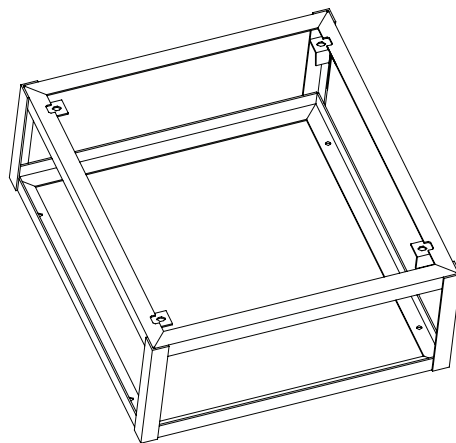
Общий вид и размеры монтажной рамы одиночного блока с нижней подачей воздуха
