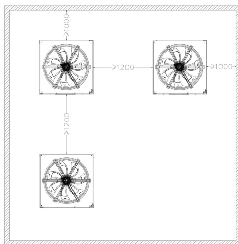
Пространство, необходимое для монтажа одиночного блока, вид сверху (ед. изм.: мм)
