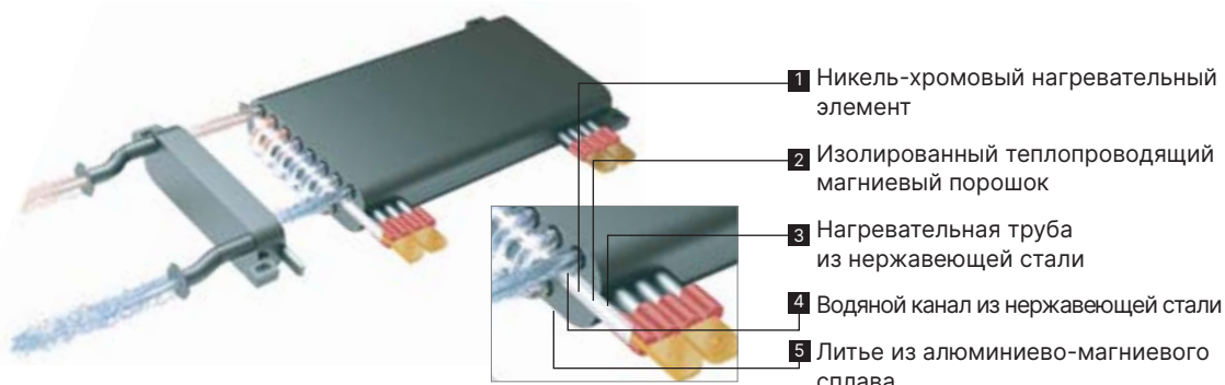
Внутренний вид котла Nobby Electro KBK
