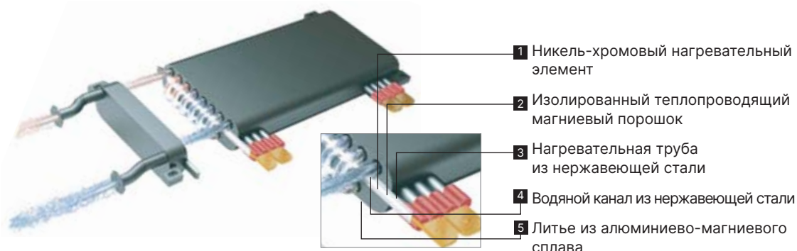
Внутренний вид котла Nobby Electro KBQ
