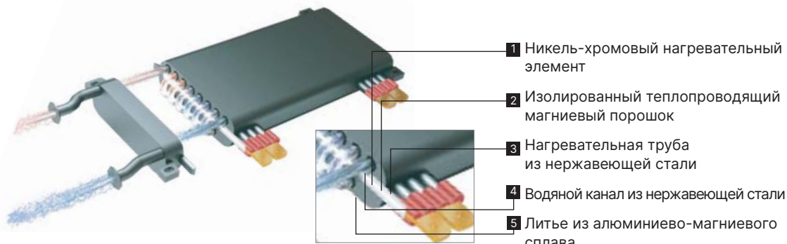
Внутренний вид котла Nobby Electro KBG
