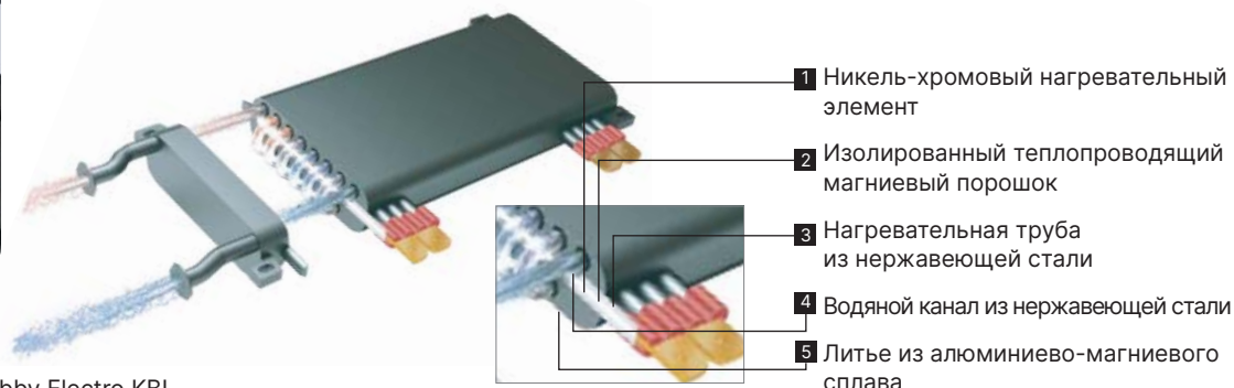
Внутренний вид котла Nobby Electro KBL
