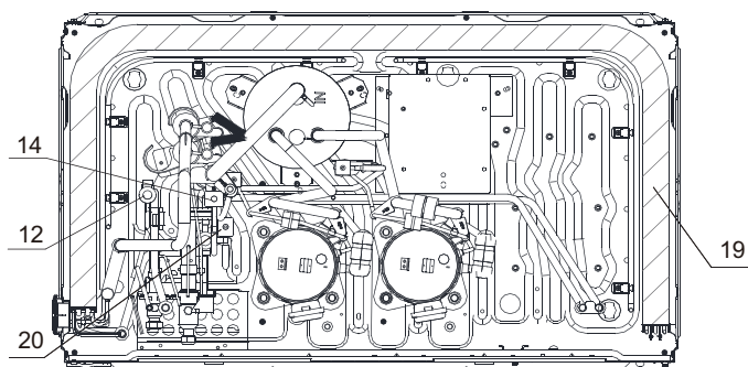
Условные обозначения № Наименование элементов 1 Компрессор 2 Сепаратор масла 3 Реле высокого давления 4 Обратный клапан 5 Датчик высокого давления 6 Вентилятор 7 Микроканальный теплообменник 8 Запорный вентиль (труба газовой линии) 9 Электронный расширительный вентиль (EEVA) 10 Порт для заправки 11 Запорный вентиль (жидкостная труба) 12 Электронный расширительный вентиль (EEVC) 13 Электронный расширительный вентиль (ЭРВ по заказу) 14 Электромагнитный клапан перепуска впрыска (SV5) 15 Клапан впрыска (SV8A/SV8B) 16 Датчик низкого давления 17 Газожидкостный сепаратор 18 Глушитель 19 Теплообменник 20 Перепускной вентиль жидкости (SV6)
