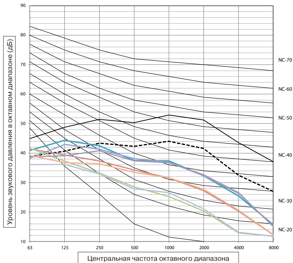
Фанкойл KFKF34H0EN1
