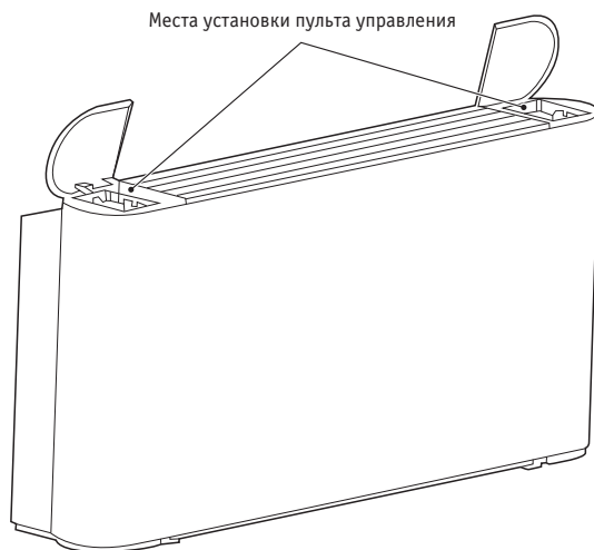
Рисунок 3-1. Место установки проводного пульта управления
