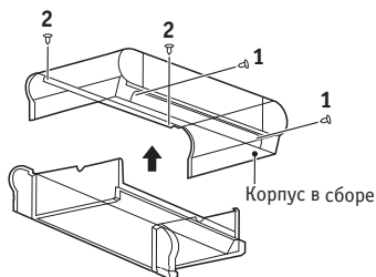
Рисунок 4-6. Снятие корпуса
