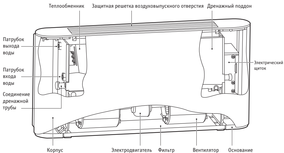
Рисунок 4-2. Изображение блока (открытого типа)
