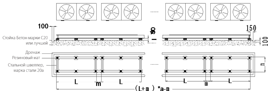
I. Схема монтажного основания из стального швеллера
