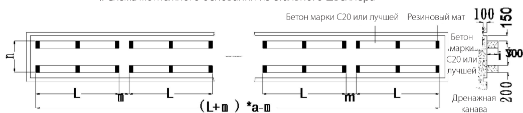
II. Схема монтажного основания из бетона
