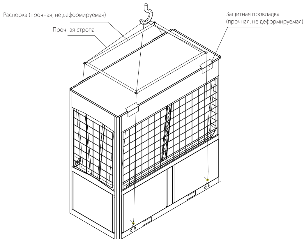
Схема строповки моделей KCRM1000HFAN3A
