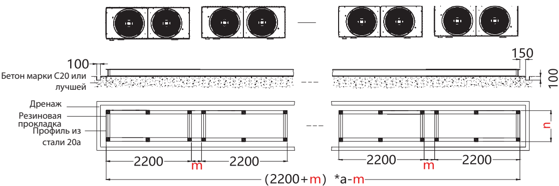
1. Схема основания из стального швеллера
