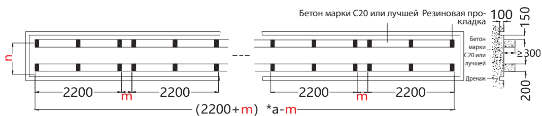
2. Схема фундамента из бетона
