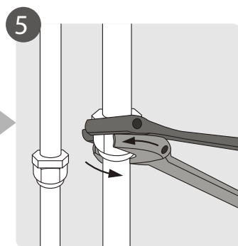
Соедините трубы
