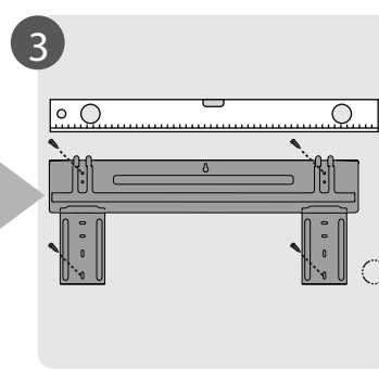
Закрепите монтажную пластину
