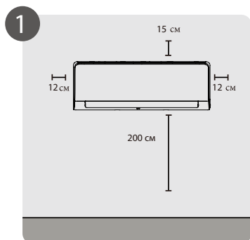
Выбрать место для установки
