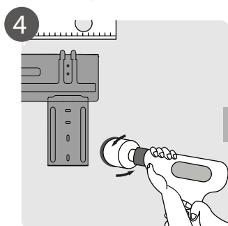
Просверлите отверстие в стене
