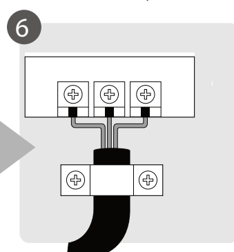
Подключите электропроводку
