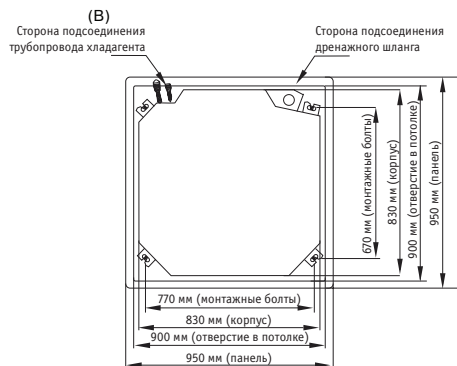
Отверстие в потолке для компактных моделей
