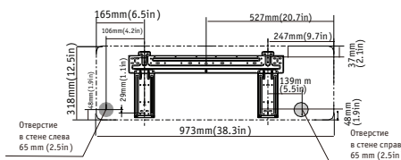
KMGA53HZRN1
