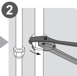
Присоедините трубы хладагента
