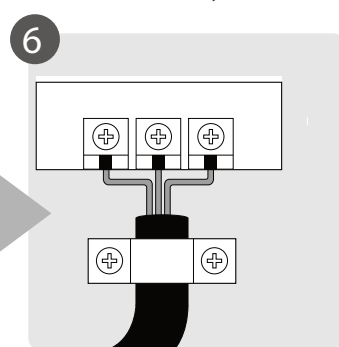
Подключите электропроводку
