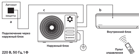
Электрический щит
