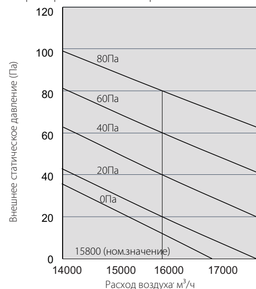
Характеристики вентилятора блока 18-20НР
