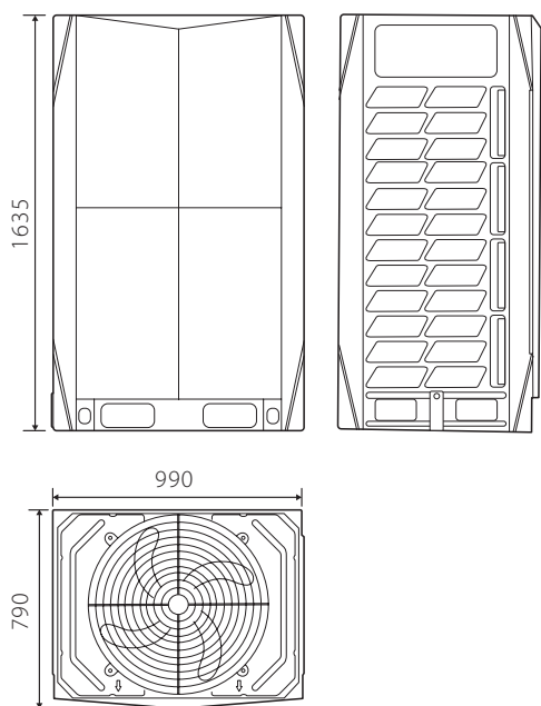
8–12 HP Ед. изм.: мм
