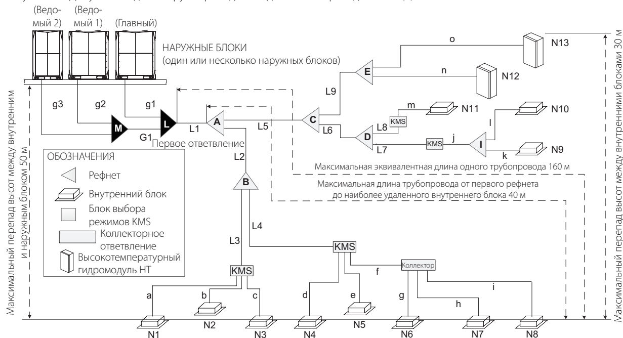
Рисунок 4-4. Допустимые длины трубопроводов хладагента и перепады высот (В)
