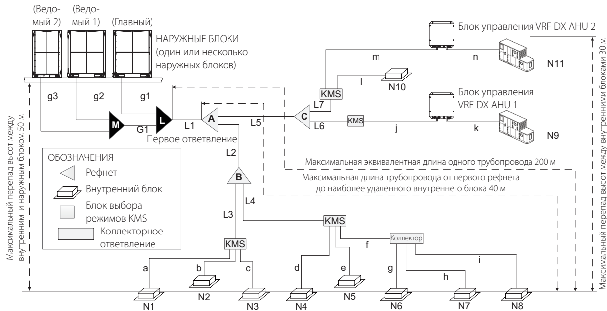
Рисунок 4-5. Допустимые длины трубопроводов хладагента и перепады высот (С)
