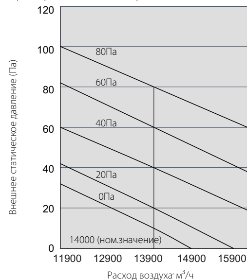
Характеристики вентилятора блока 16НР
