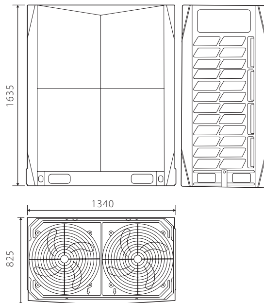
14–20 HP Ед. изм.: мм
