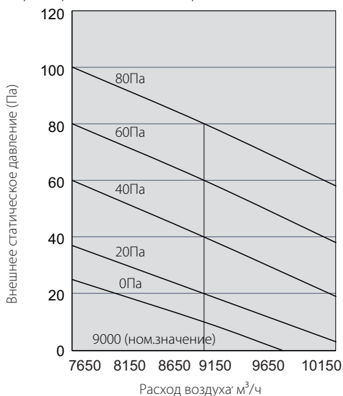
Характеристики вентилятора блока 10НР
