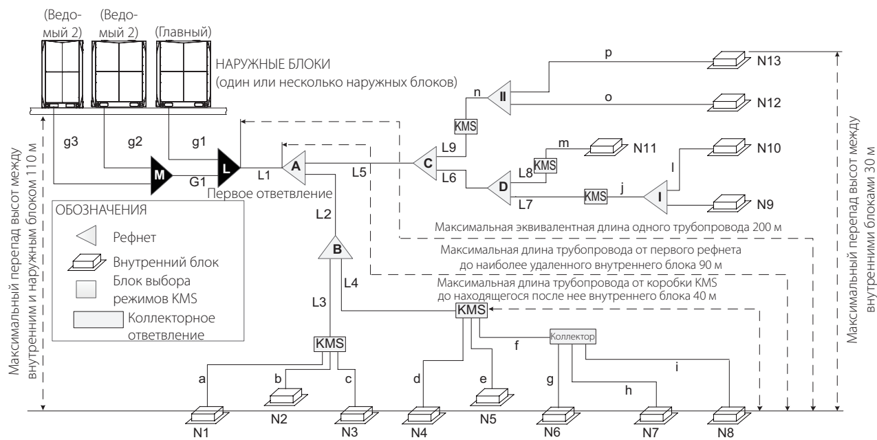
Рисунок 4-2. Допустимые длины трубопроводов хладагента и перепады высот (А)
