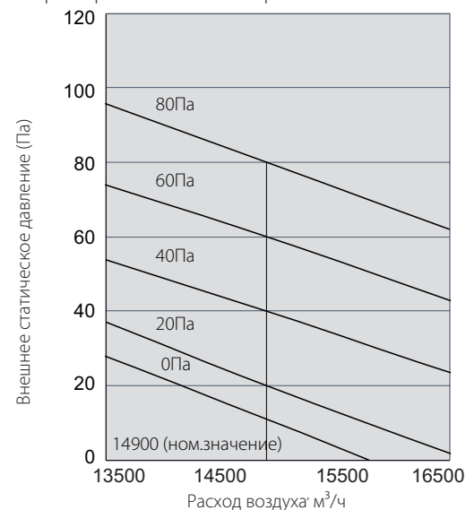
Характеристики вентилятора блока 18-20НР
