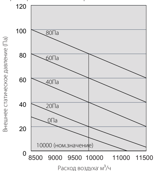
Характеристики вентилятора блока 12НР
