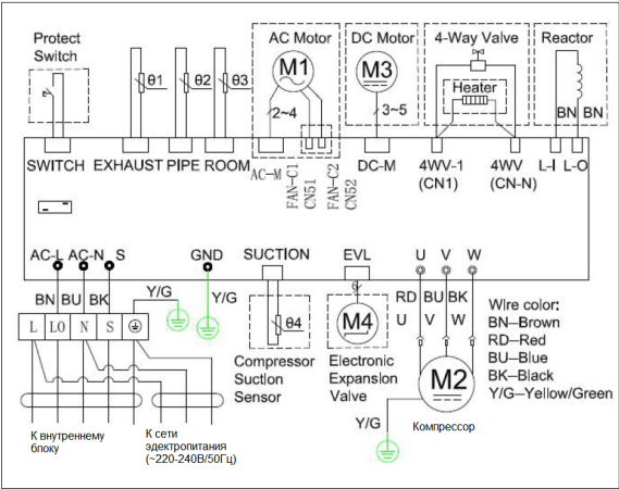
Схема электрическая наружных блоков
