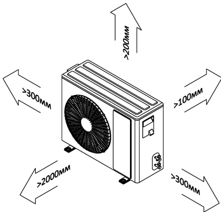
Установочные размеры наружных блоков
