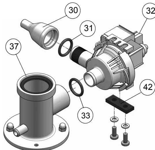
Шламоотводящий насос
