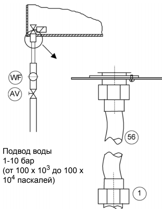
Подключение 3/4"
