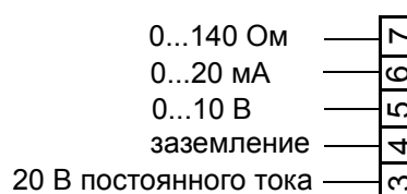
Соединительные клеммы для управляющих сигналов
