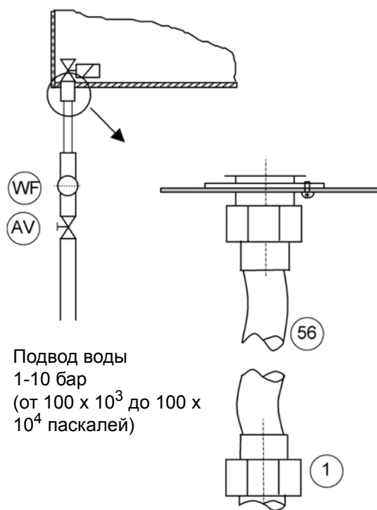
Подключение 3/4"
