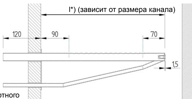
Горизонтальный монтаж в канале
