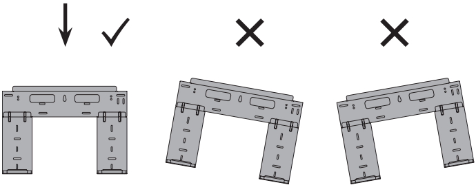
Правильное положение монтажной панели
