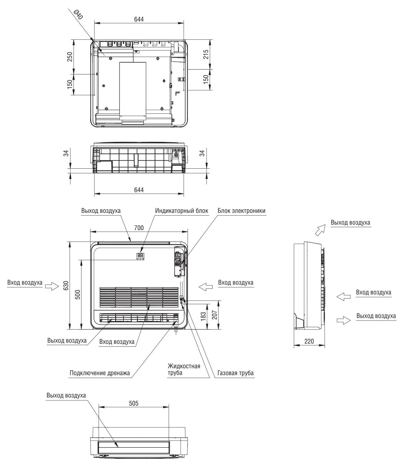
Блоки консольного типа, модели 9/12
