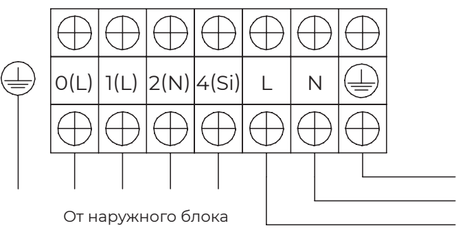
Клеммный терминал наружного блока
