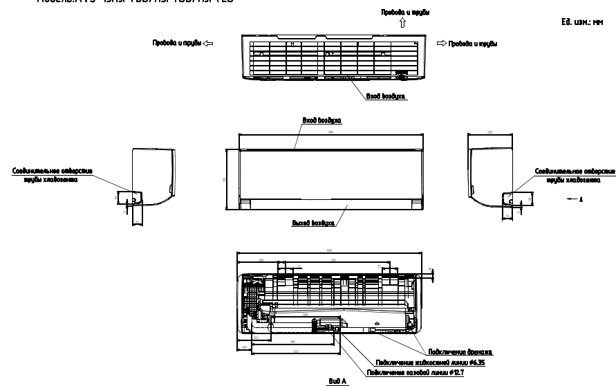
Модель: AVS-15HJTDD/H3FTDD/HJFTED
