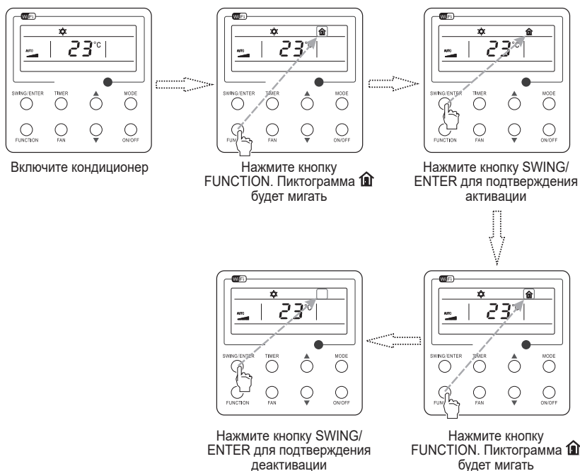
Рис. 18. Активация функции дежурного нагрева +8 °C
