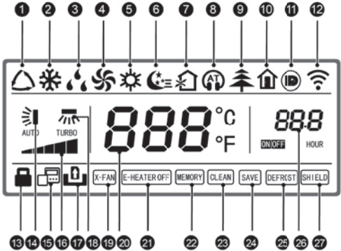
Рис.2 ЖК-дисплей проводного пульта
