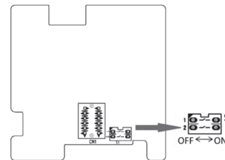
Рис. 28. Схема DIP-переключателей
