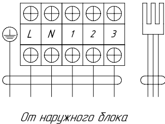
Клеммный терминал внутреннего блока
