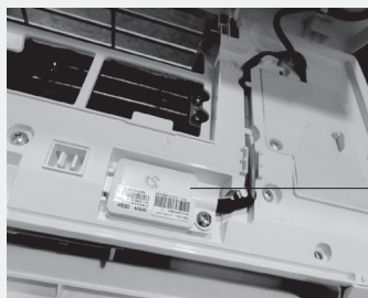
модуль Wi-Fi
