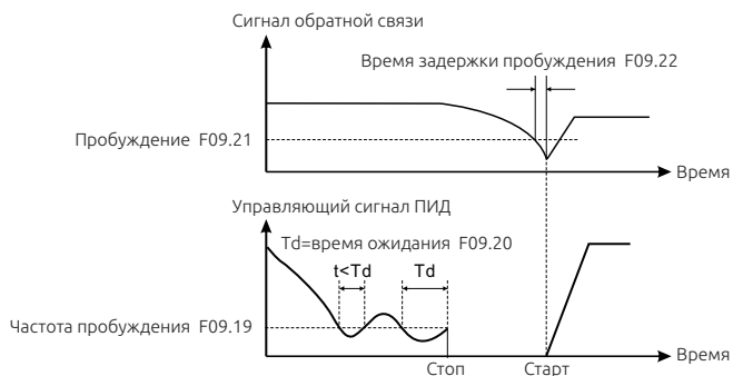
График режимов ожидания-пробуждения ПИД регулятора
